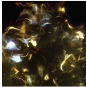
Glia
